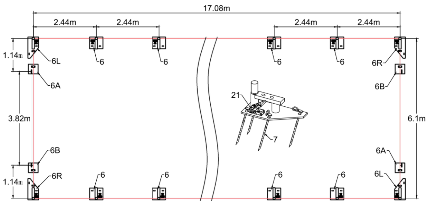
Obrázok 2. Základná doska
