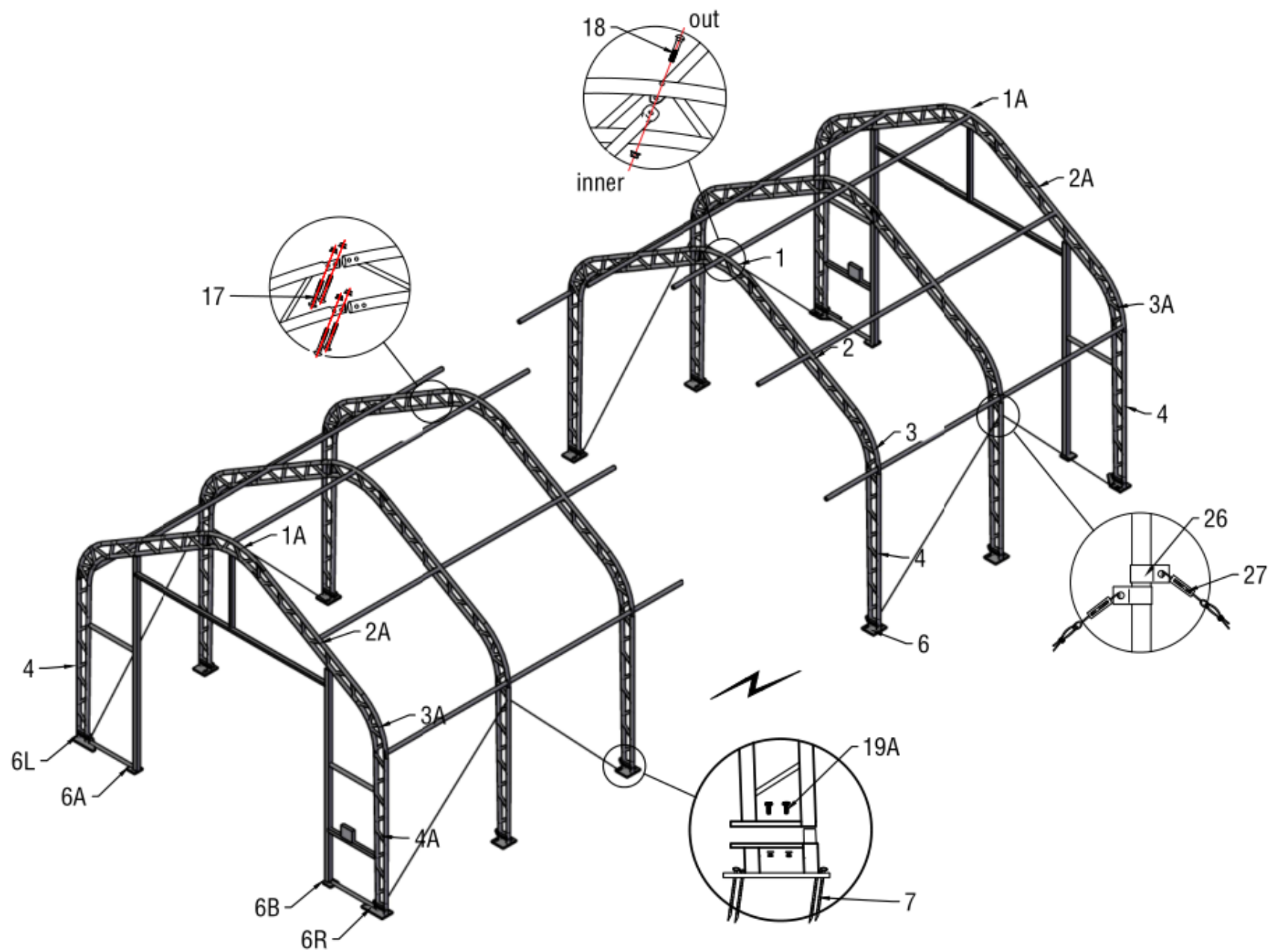
Obrázok 1: Náčrt rámu
