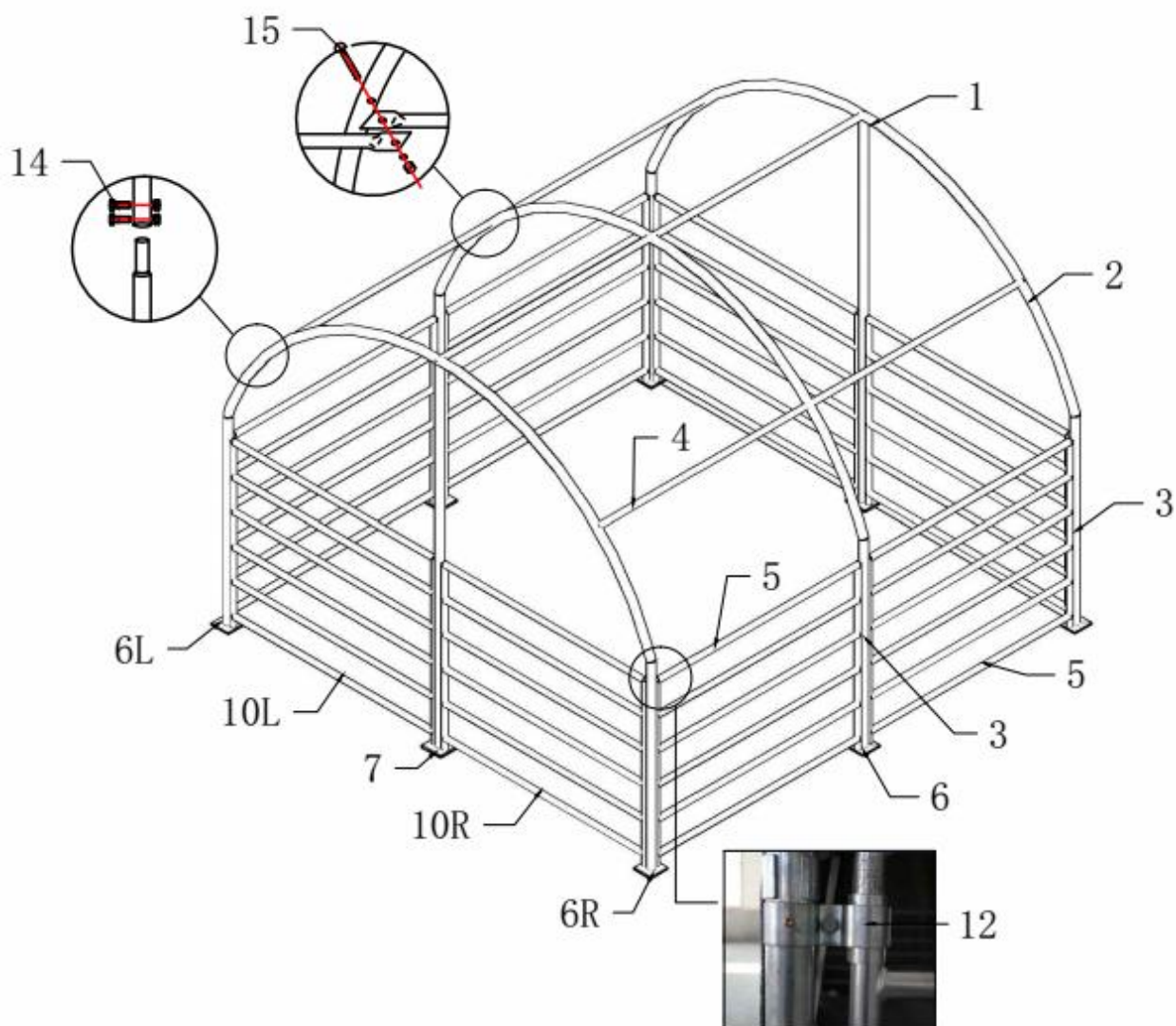
Obrázok 1: Náčrt oceľového rámu
